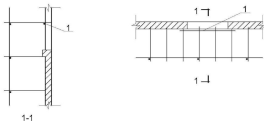
图 6.5.3 单排脚手架过窗洞构造
