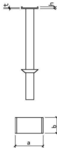
图 3 可调托撑构造图
