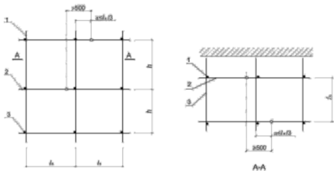
(a) 接头不在同步内（立面）
