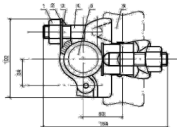
图 6 直角扣件
